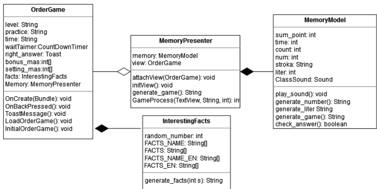
Рисунок 15 – Диаграмма классов для игры из категории «Память»
