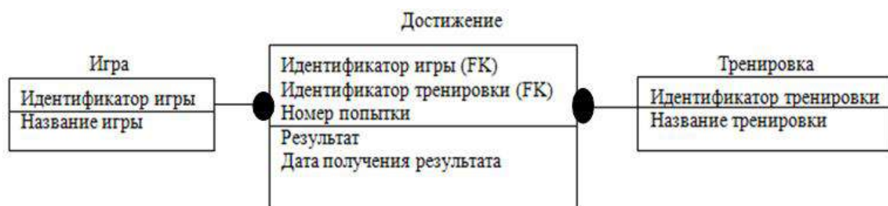
Рисунок 21 – Логическая схема базы данных
