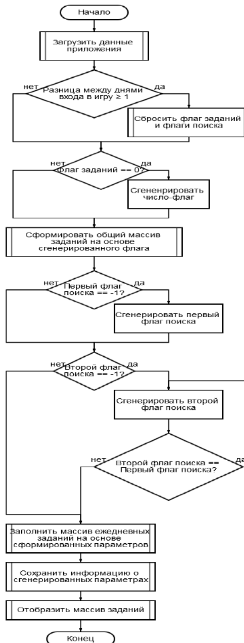
Рисунок 18 –Алгоритм генерации ежедневных заданий
