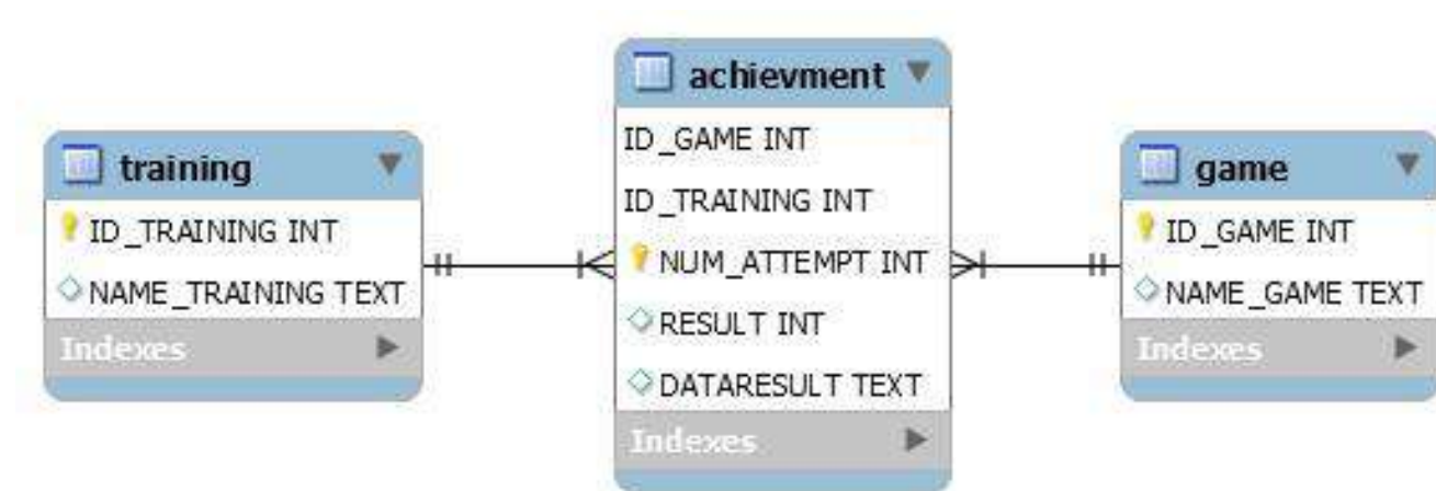
Рисунок 22 – Физическая схема базы данных
