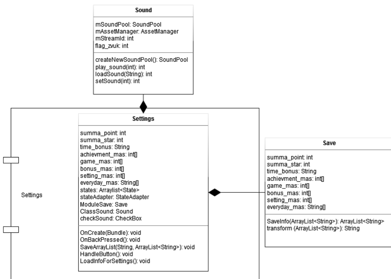
Рисунок 8 – Диаграмма классов модуля для работы с настройками
