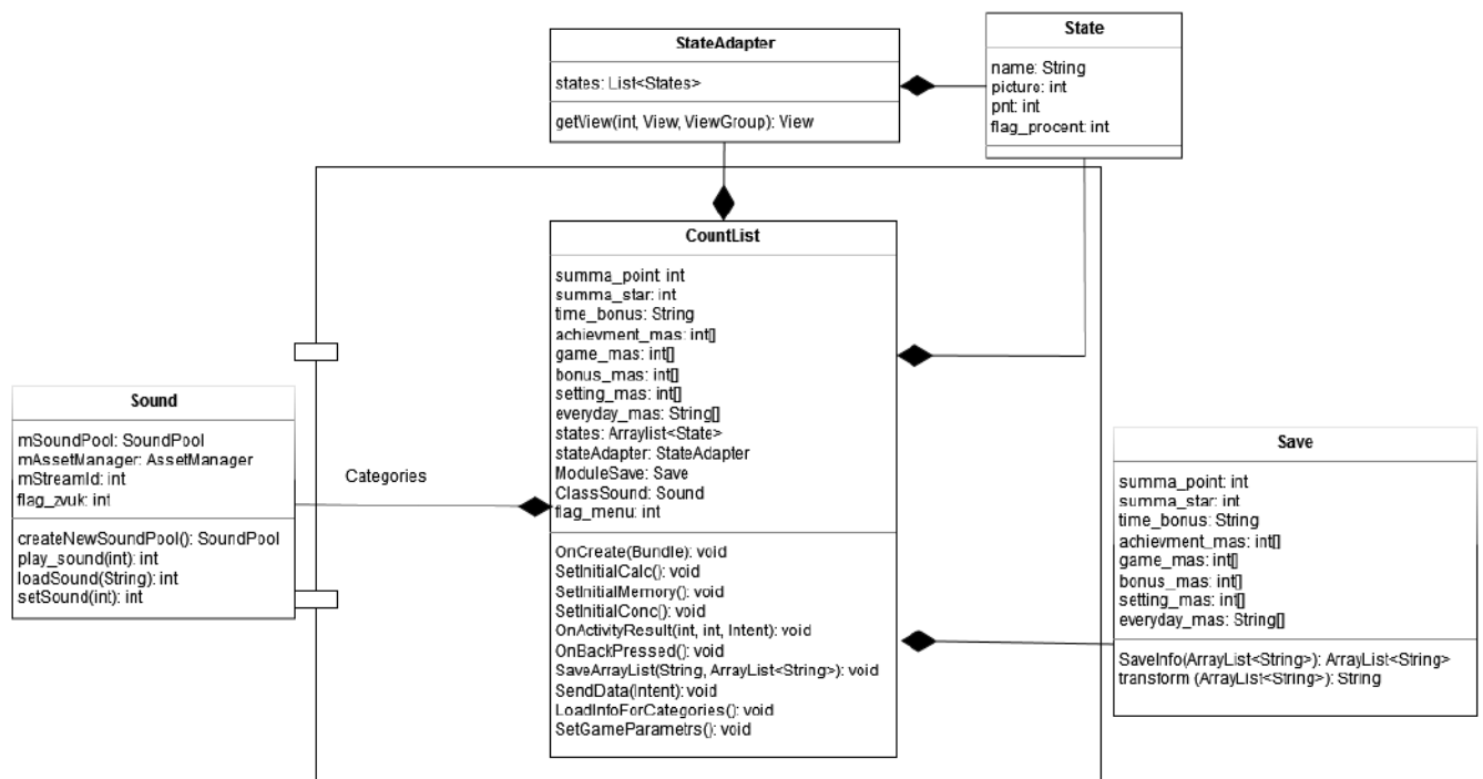
Рисунок 12 – Диаграмма классов модуля для работы с категориями развивающих игр
