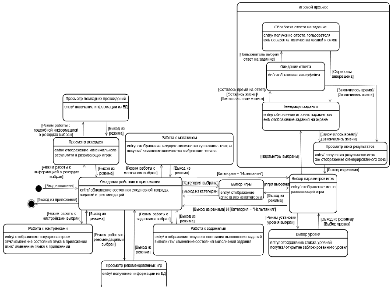
Рисунок 6 – Состояния разрабатываемого мобильного приложения
