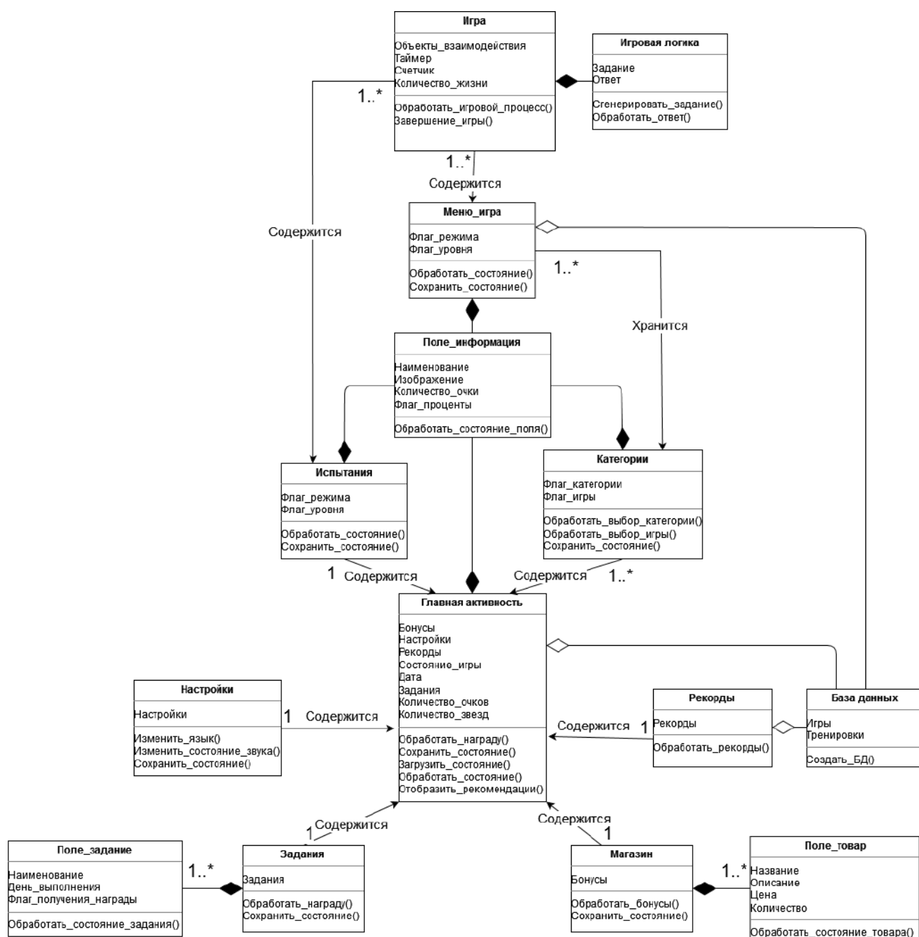
Рисунок 5 – Концептуальная модель разрабатываемого приложения
