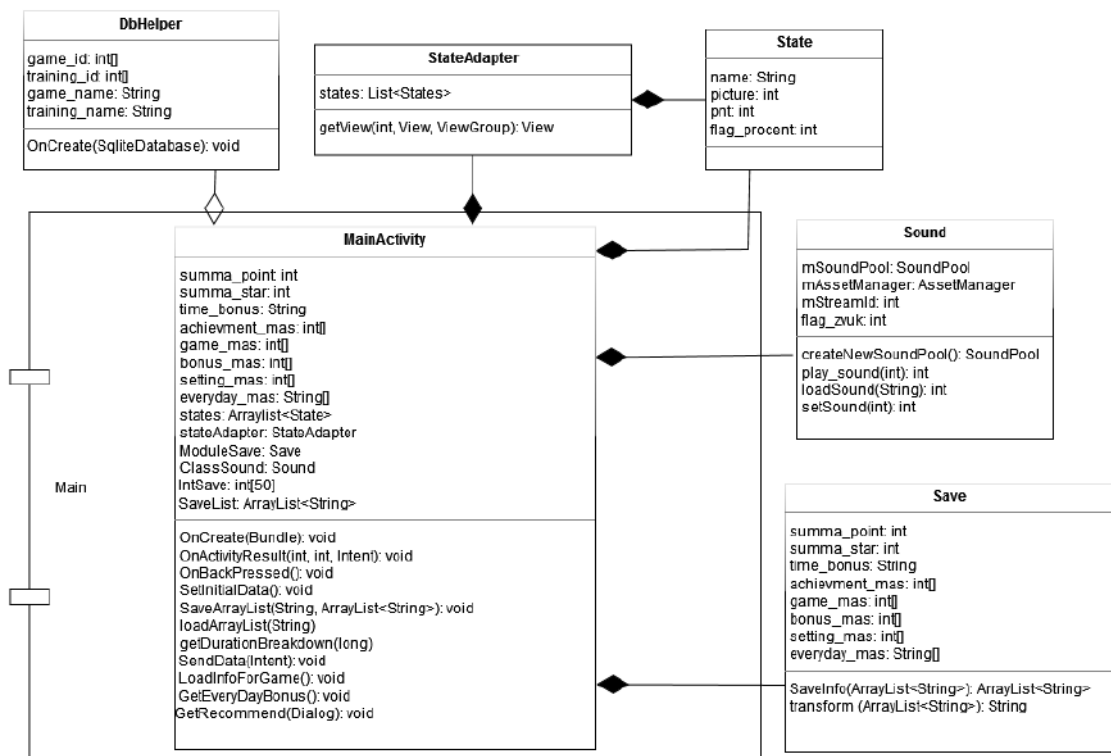
Рисунок 7 – Диаграмма классов главного модуля
