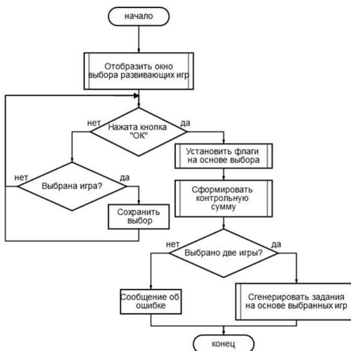
Рисунок 19 –Алгоритм самостоятельного формирования тренировки типа «Испытание»
