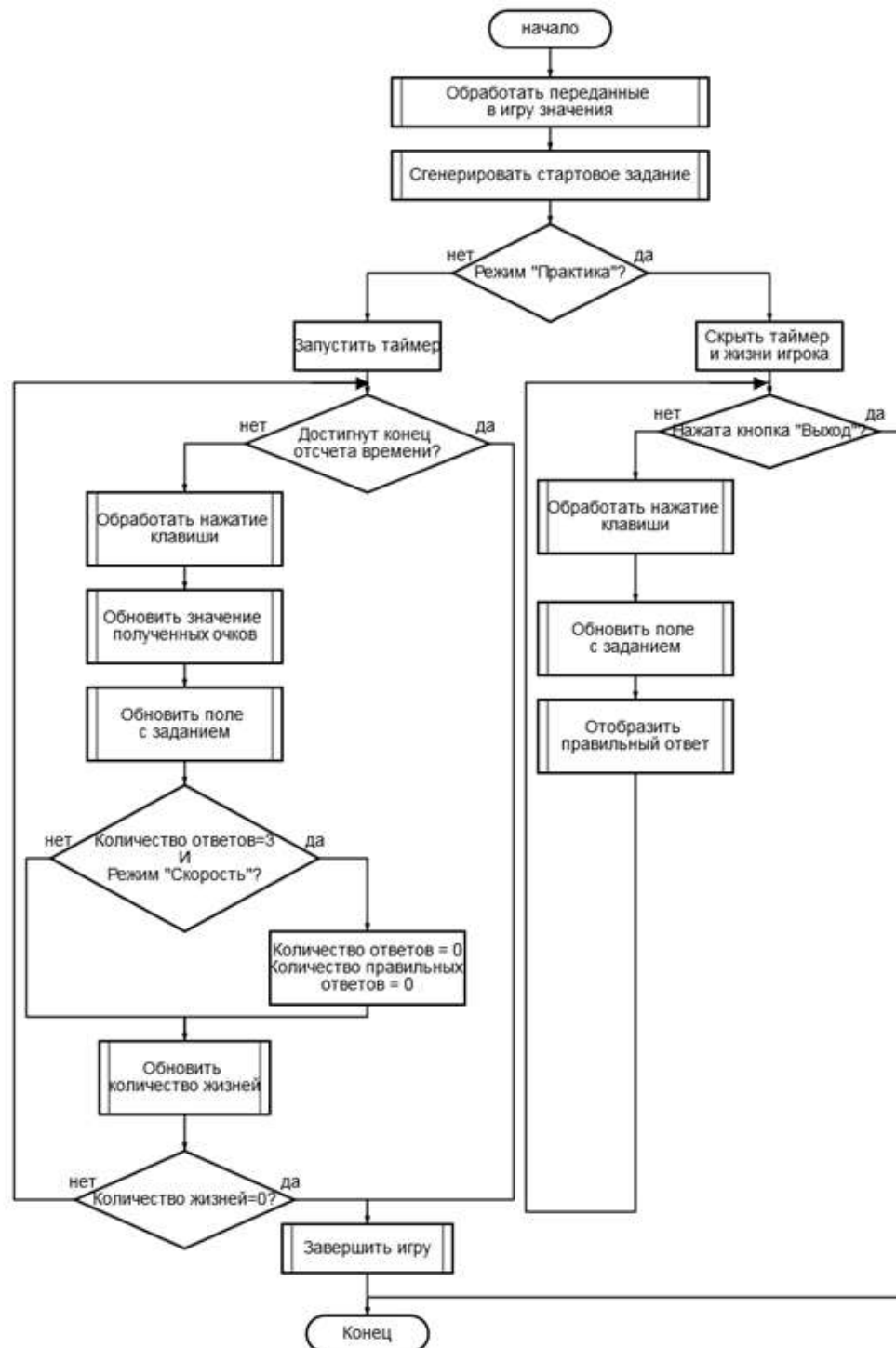
Рисунок 17 – Общий алгоритм большинства развивающих игр
