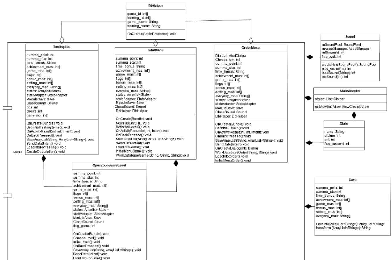
Рисунок 13 – Диаграмма классов модуля для работы с меню развивающих игр
