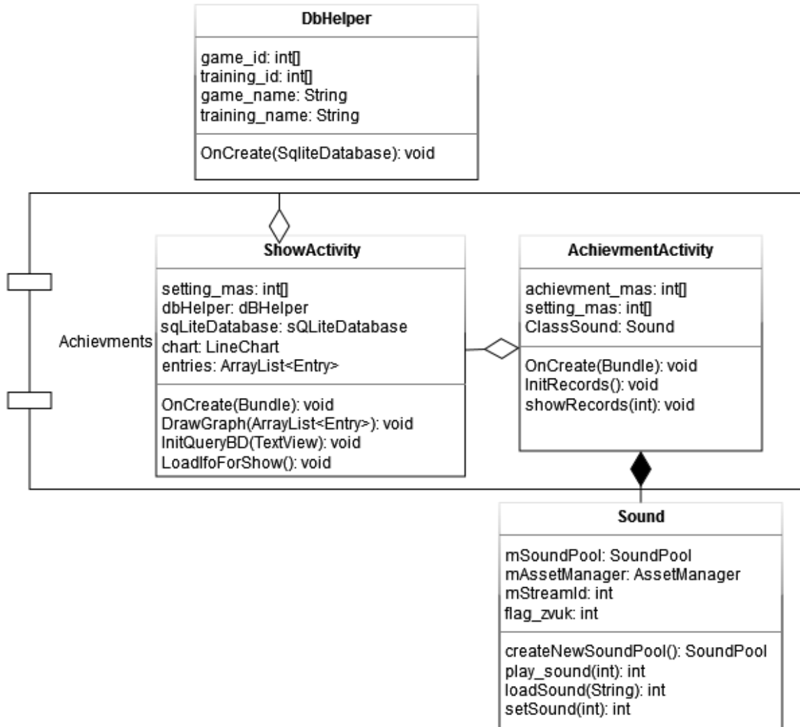
Рисунок 9 – Диаграмма классов модуля для отображения рекордов
