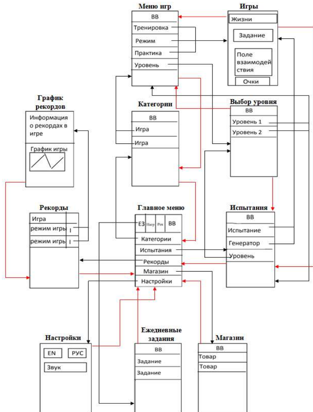
Рисунок 20 – Схема экранов разрабатываемого приложения
